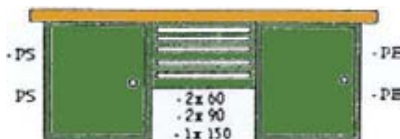
Tavolo con 2 T27 con porta H. 750 mm. 2 piani spostabili e 2 piani estraibili, 1 T24 con 5 cassetti.
