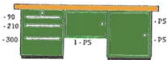
Tavolo con 1 T25 con tre cassetti, 1 T25 con porta e 2 piani, 1 T24 con 1 piano, 2 zoccoli H. 130 mm.
