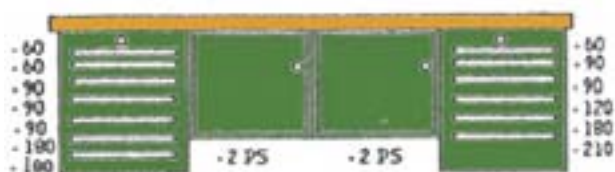
Tavolo con cassetteria 2 T27 a 13 cassetti, 2 T 25 con porta H.600 mm 4 piani spostabili
