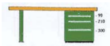
Tavolo con cassetiera T25 a 3 cassetti, gamba H 830 mm, zoccolo H.130 mm
